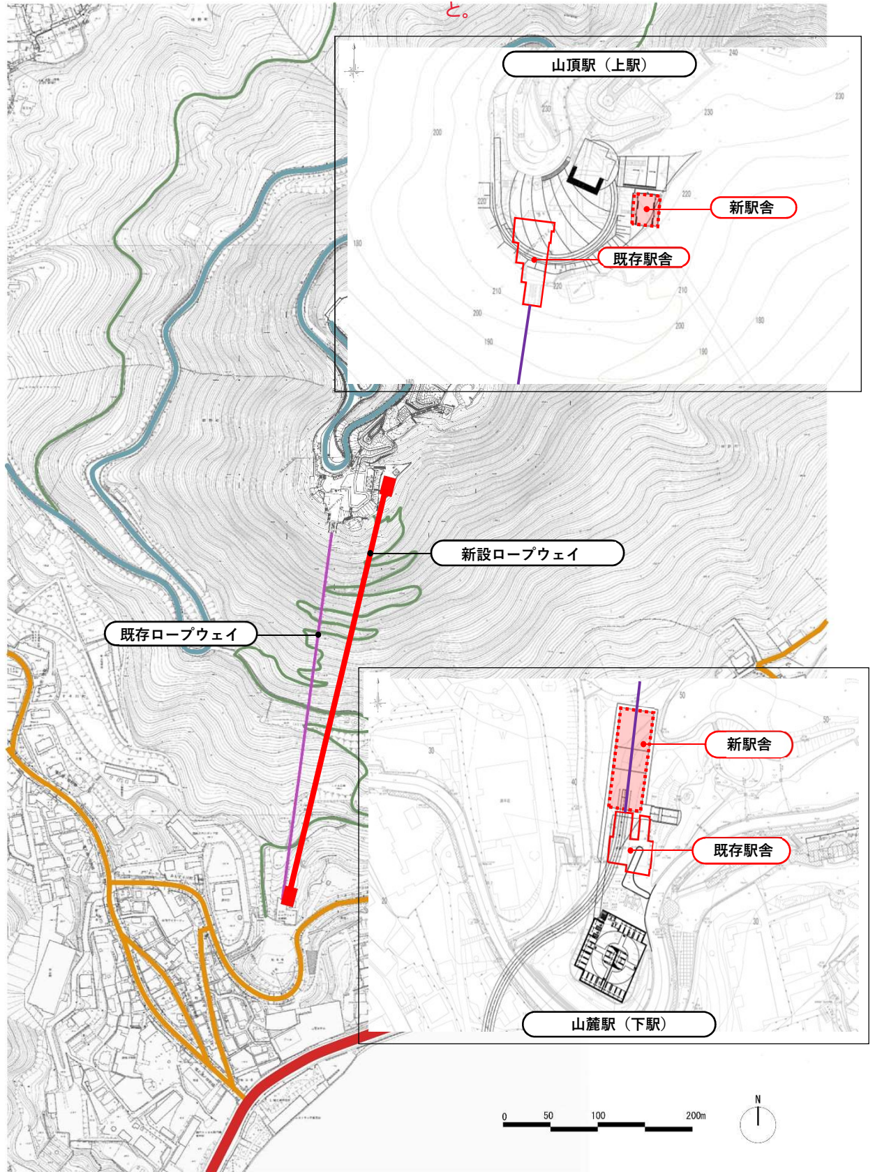
別図1 配置図
