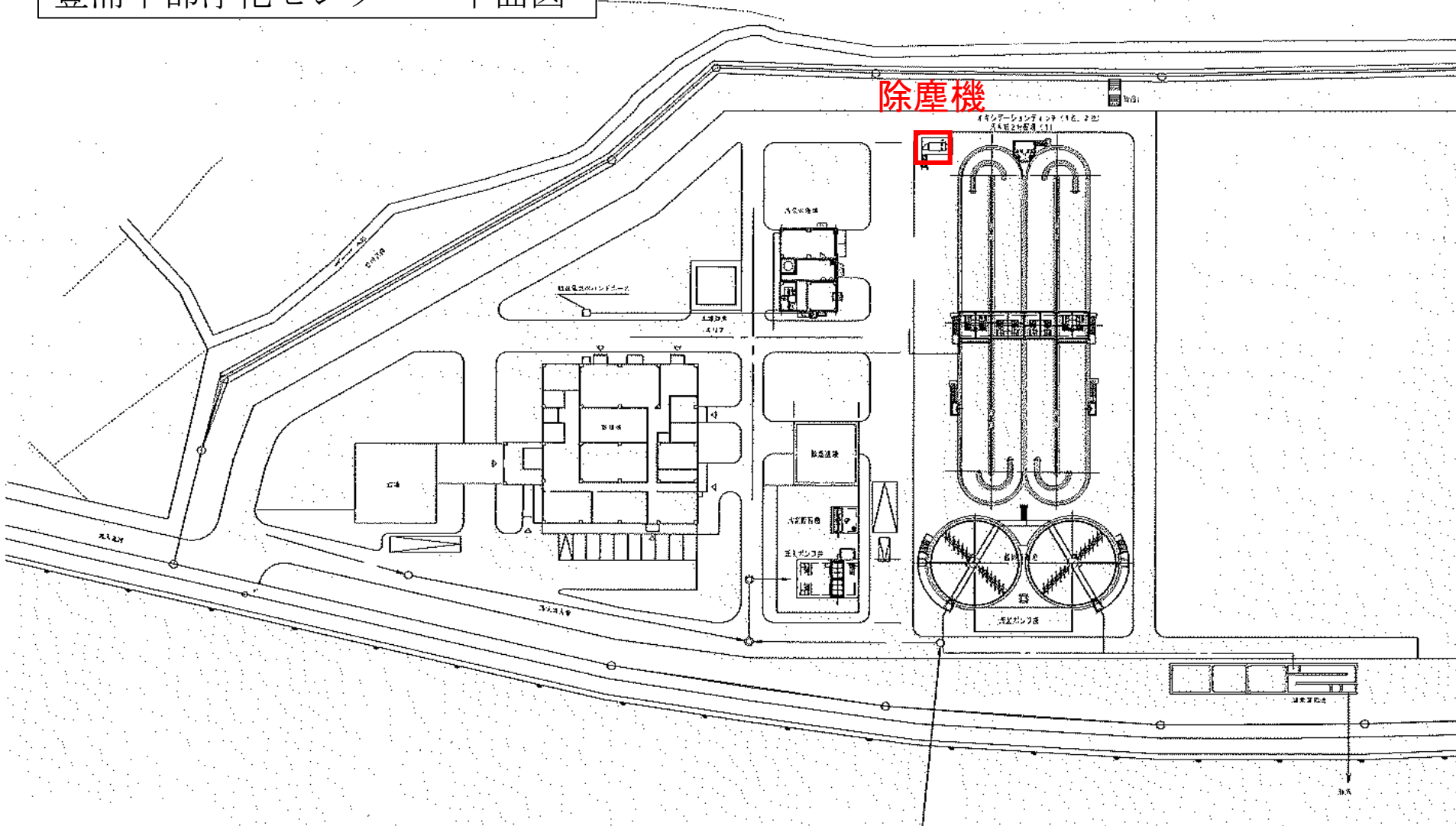
豊浦中部浄化センター 平面図
