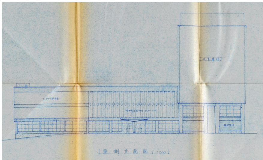
東側立面図
