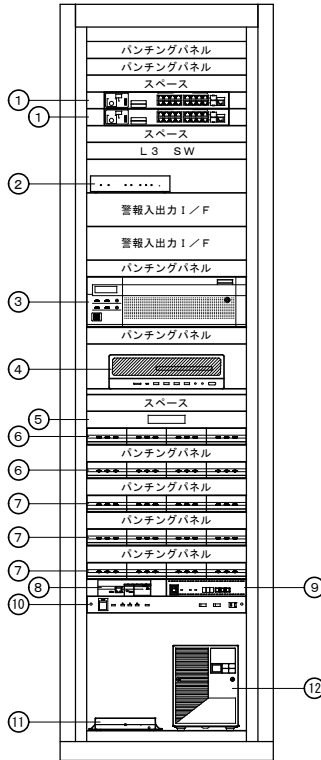
改修後機器収納図 (赤間町駐車場機器収納架)
