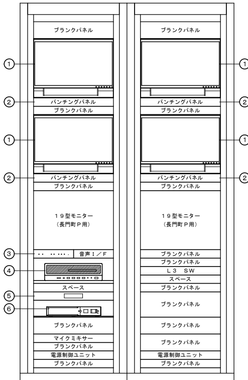
改修後機器収納図 (細江町駐車場機器収納架)
