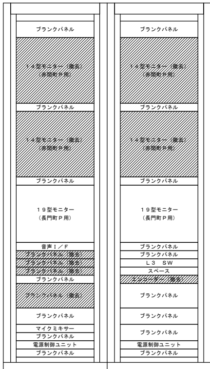
撤去機器図 (細江町駐車場機器収納架)
