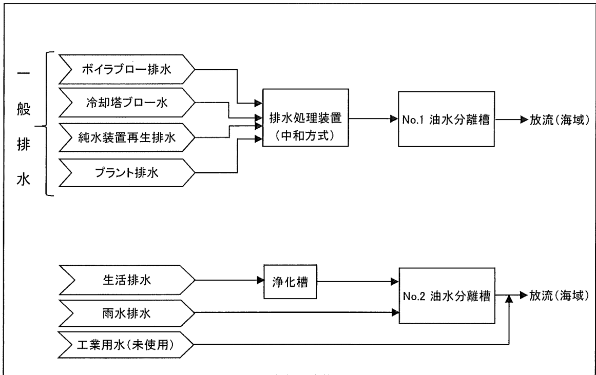
排水フロー
