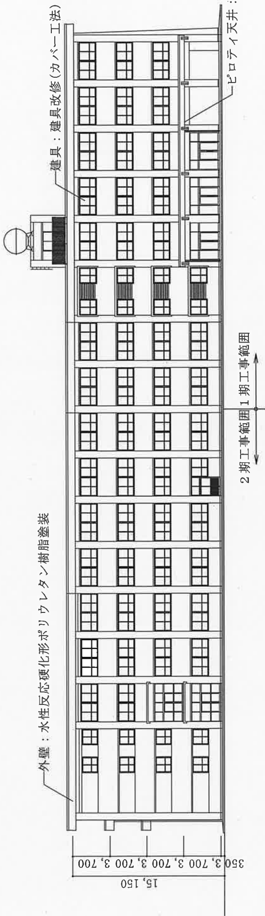
北側立面図
