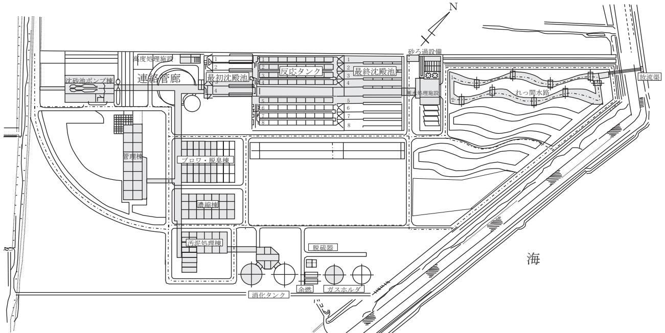
山陽終末処理場配置図
