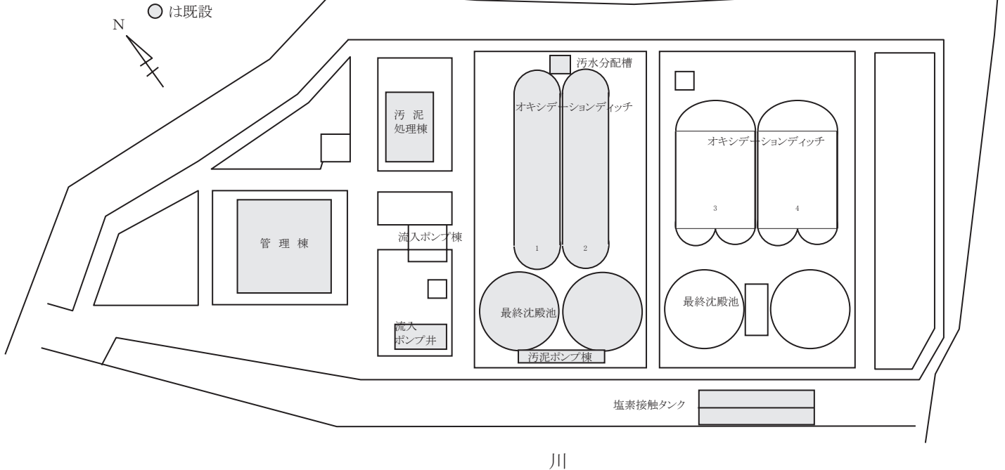
豊浦中部浄化センター配置図
