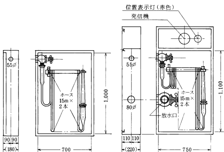
図2-3 屋内消火栓箱
