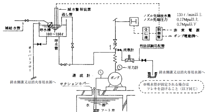
図2-2 標準加圧送水装置例
