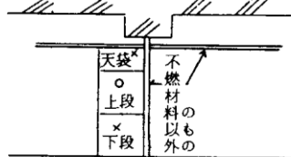
天井裏に感知器がある場合で押入等の壁面が不燃材料以外のもの
