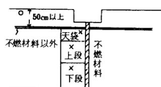
天井裏に感知器がない場合
