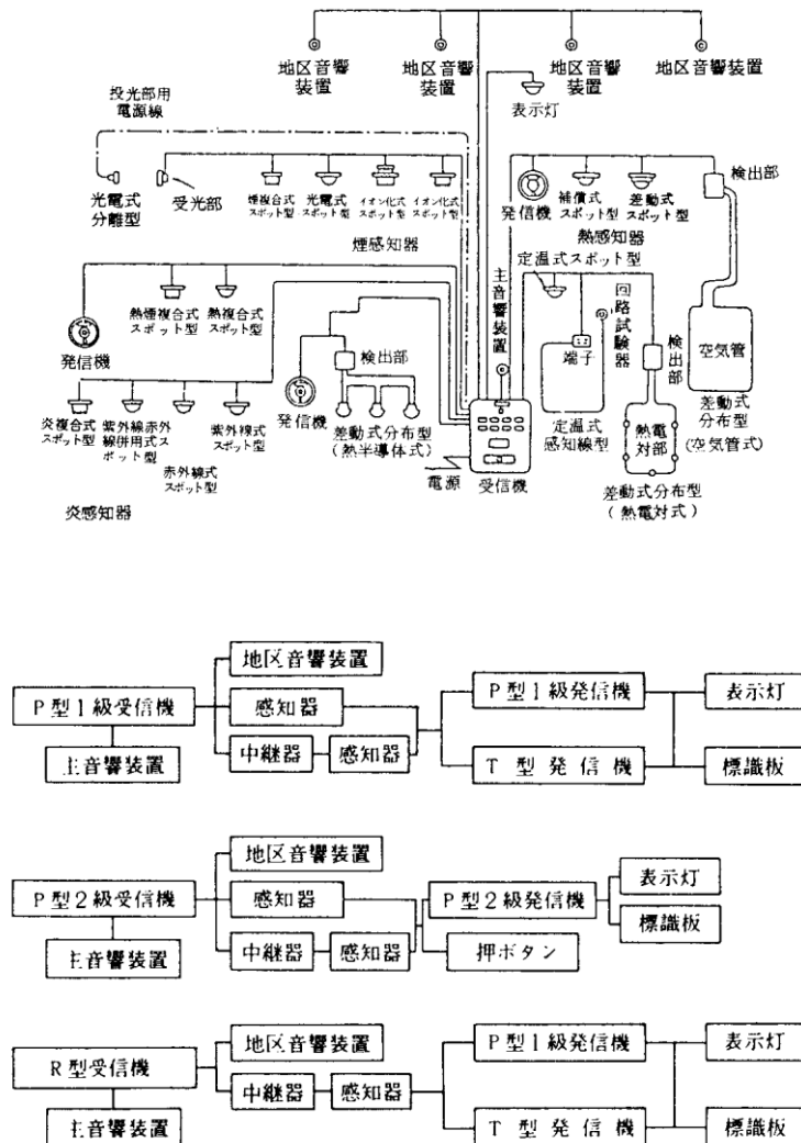
図10-1 自動火災報知設備の構成図例
