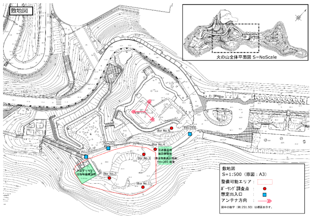
敷地図
