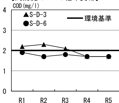
【周防灘のCODの経年変化】
