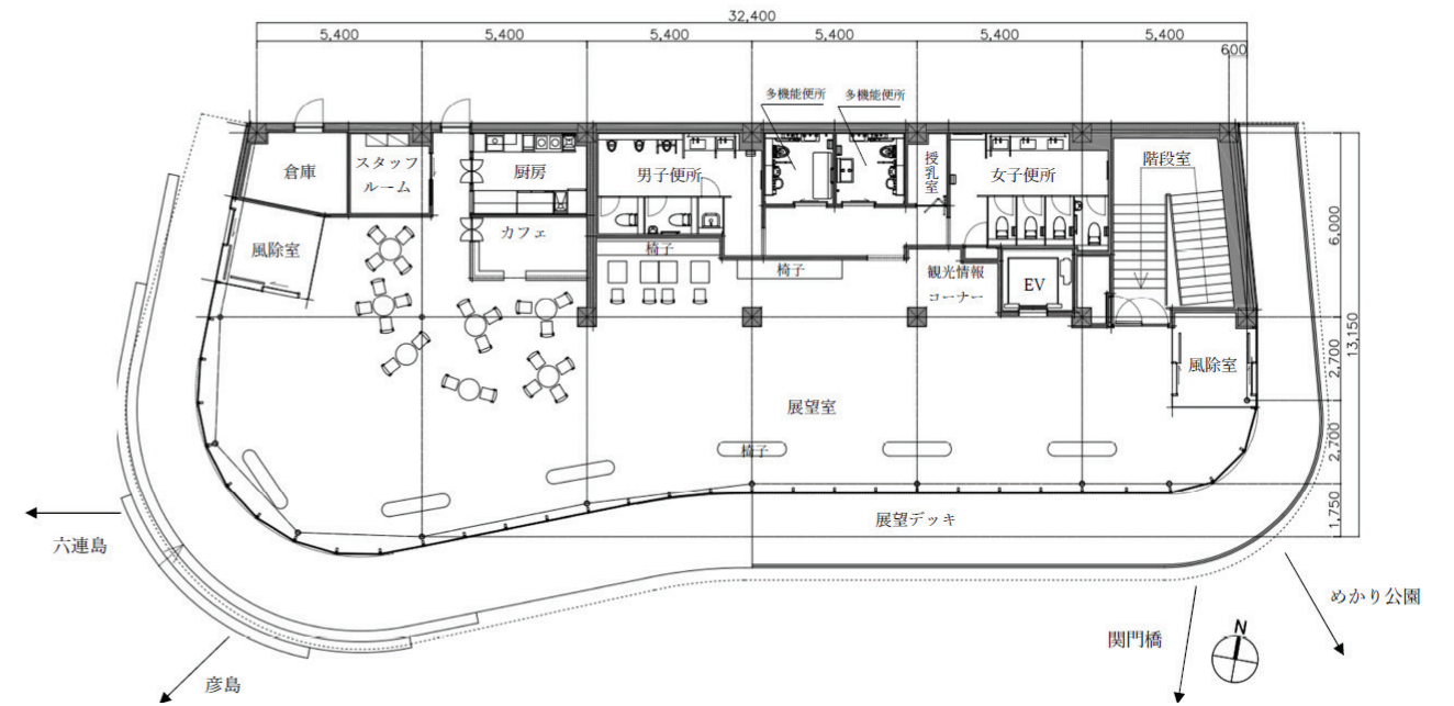
屋内展望施設レイアウト(案)
