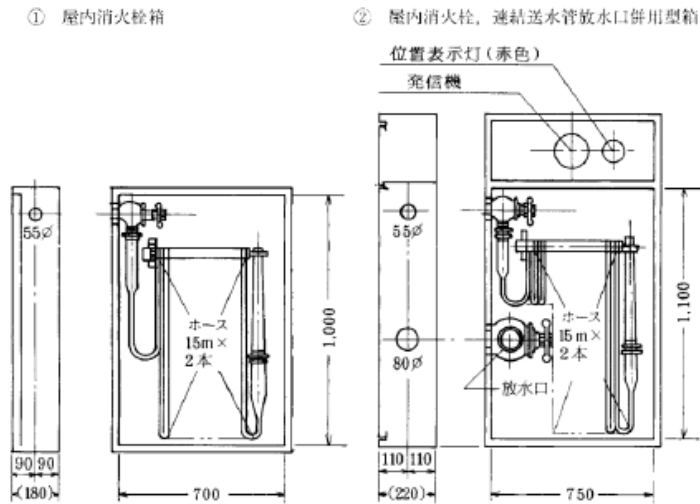
図2-3 屋内消火栓箱
