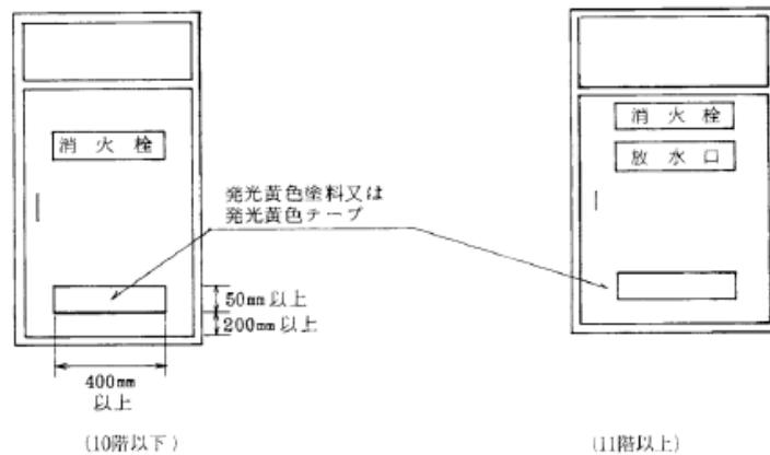
③ 屋内消火栓、連結送水管放水口併用型 ボックス表面
