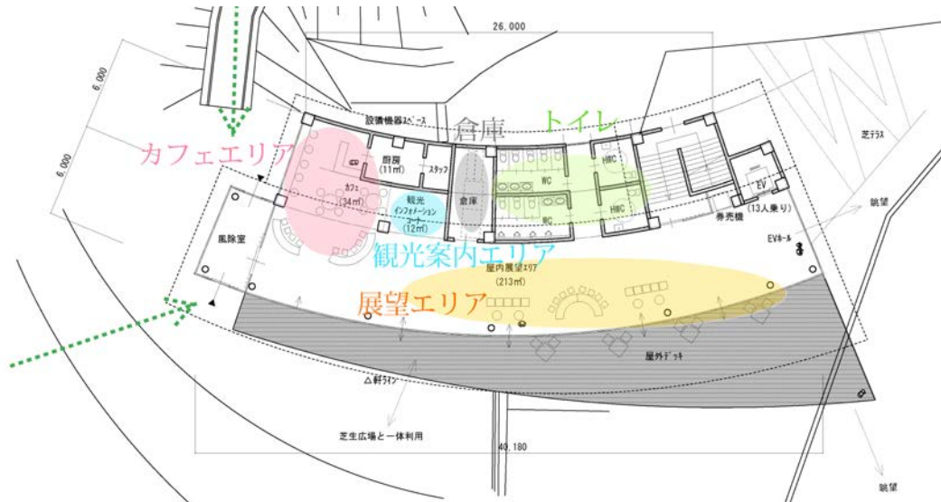
屋内展望施設兼パルスゴンドラ駅舎平面図(案)
