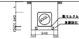
根切り1500H未満 重圧管断面図 S:1/50
