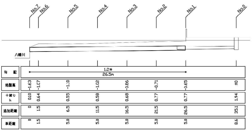
縦断面図 S:1/200
