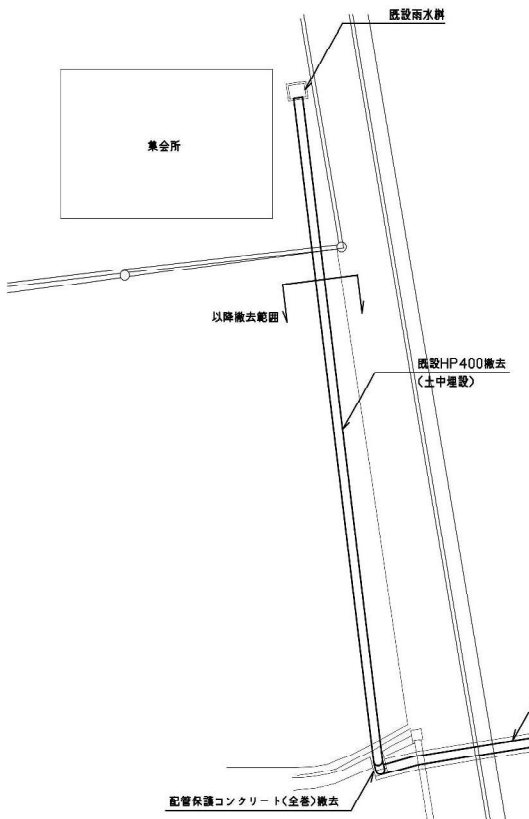
改修前平面図 S:1/200
