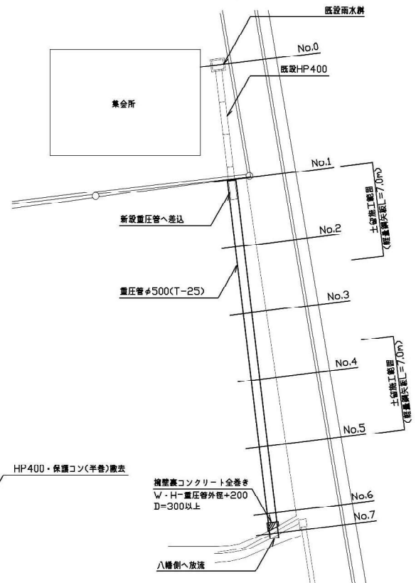
改修後平面図 S:1/200
