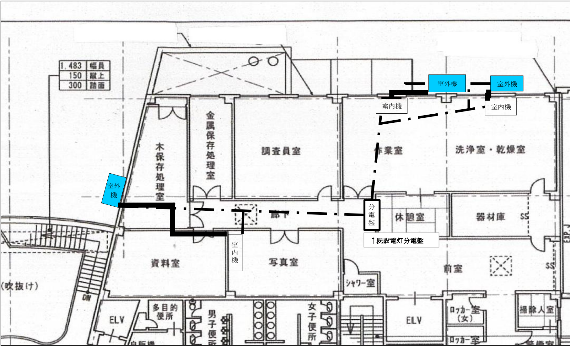
空調機・配管等設置イメージ図
