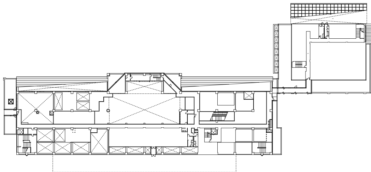
2階平面図
