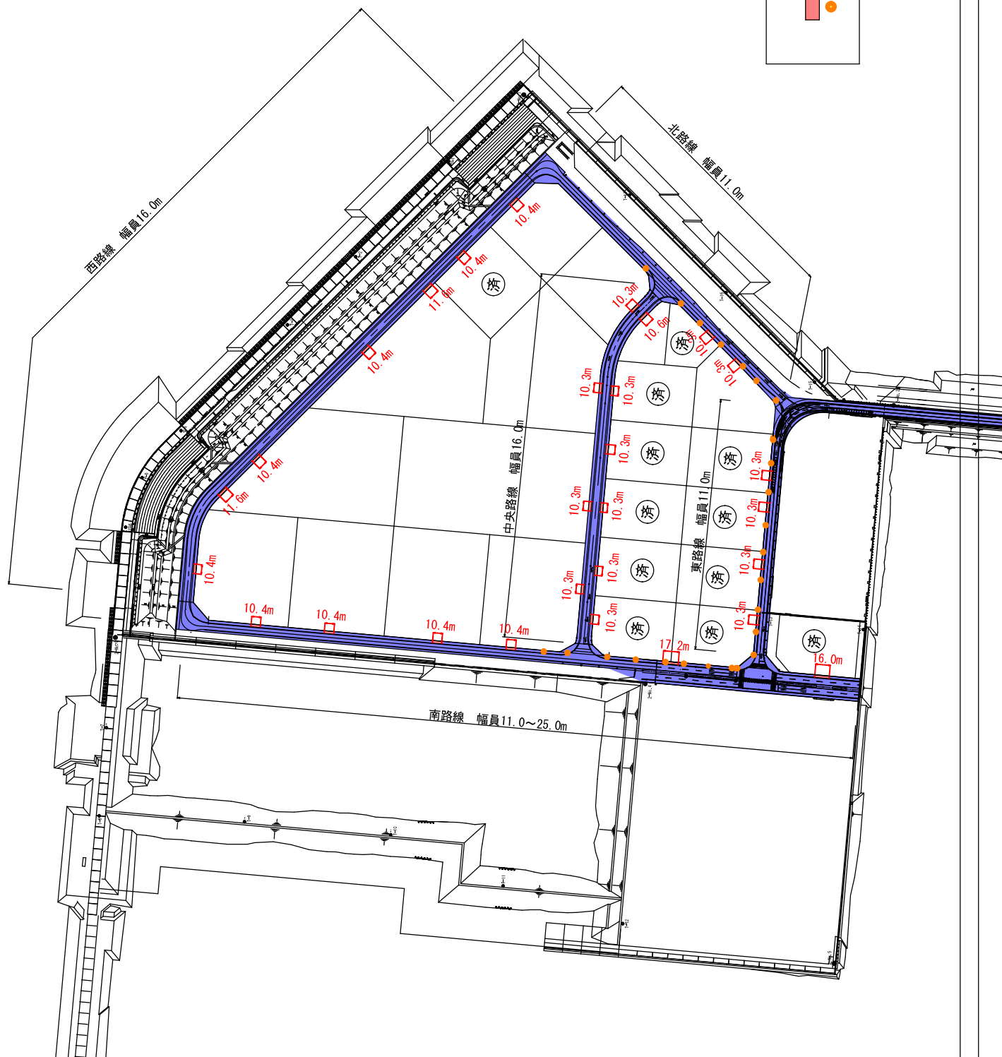
全体平面図 S = 1:4,000
