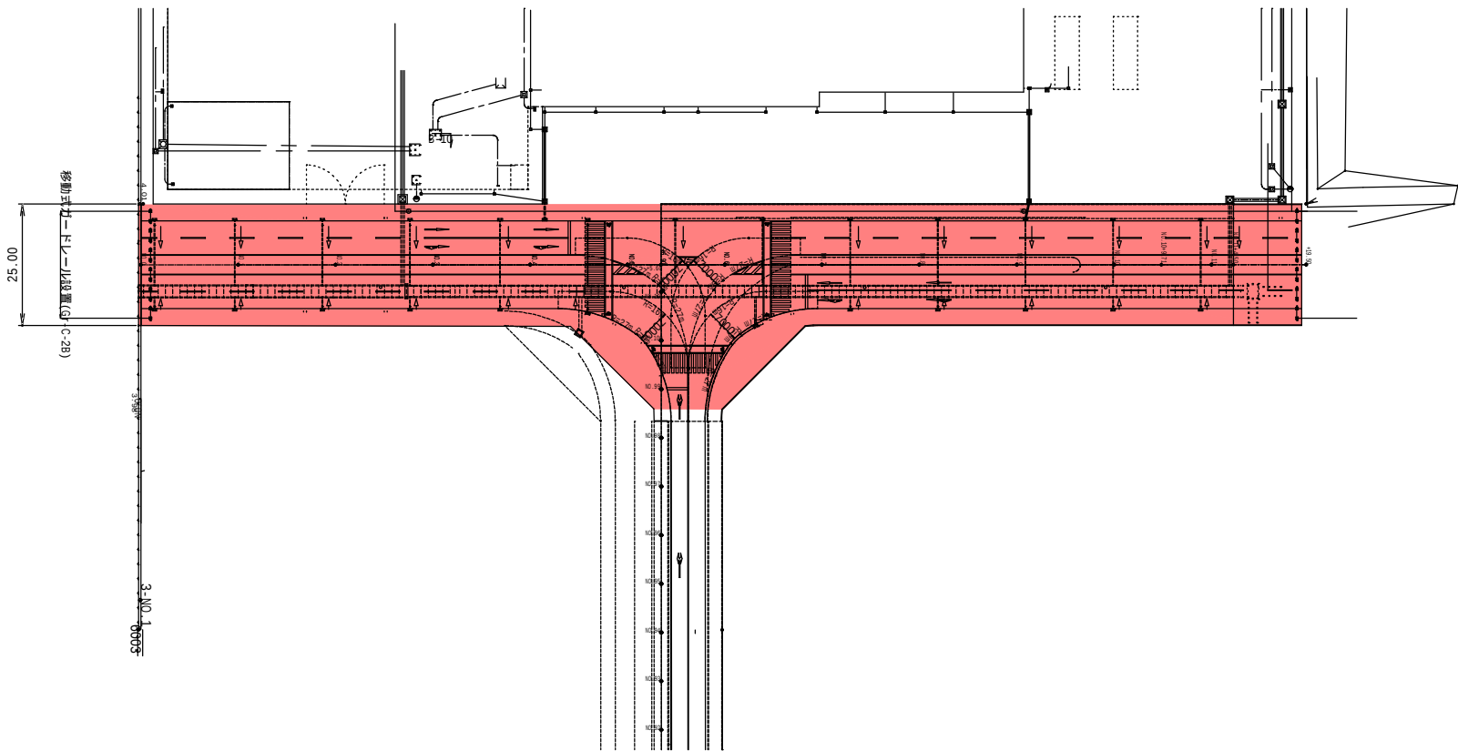
平面図 (南路線-S-2)
