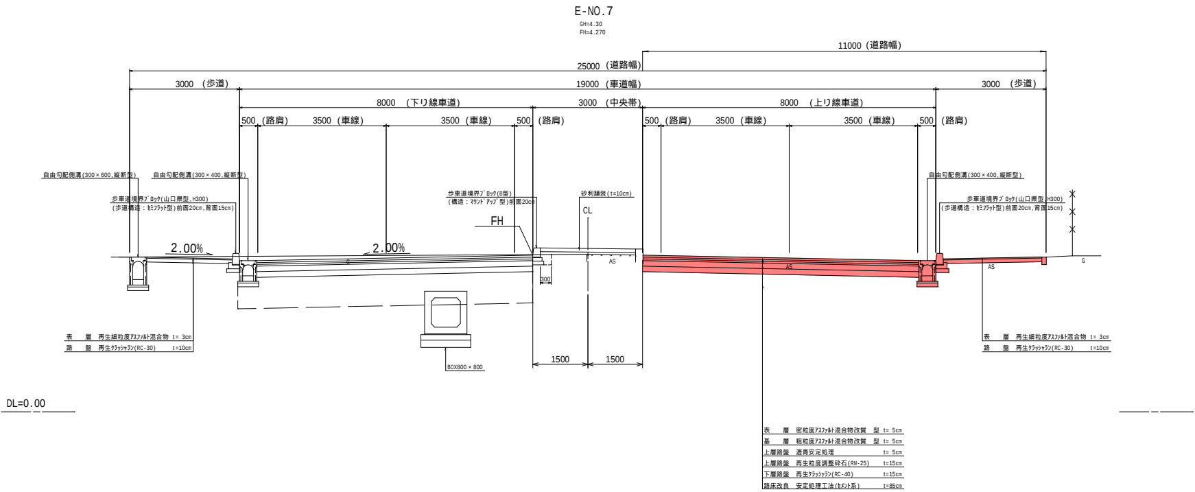
標準横断図 (東路線-E)
