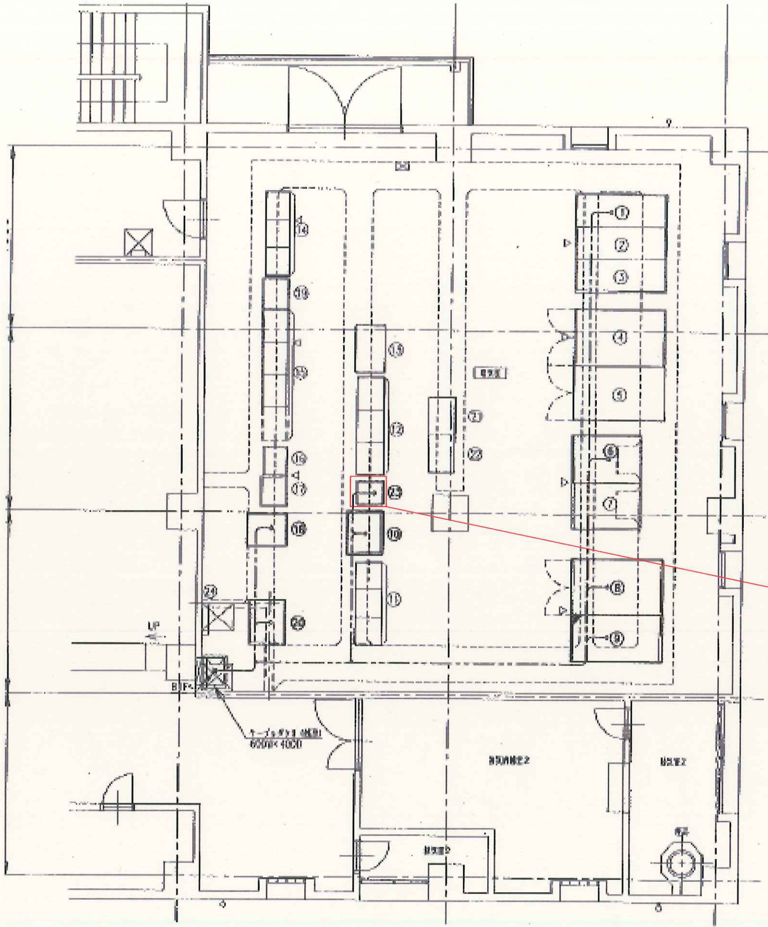
汚泥処理棟3F電気室 平面図
