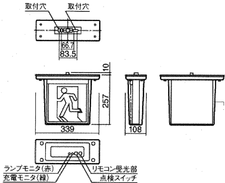
誘導灯B級B.L形片面（天井吊下げ型）参考図
