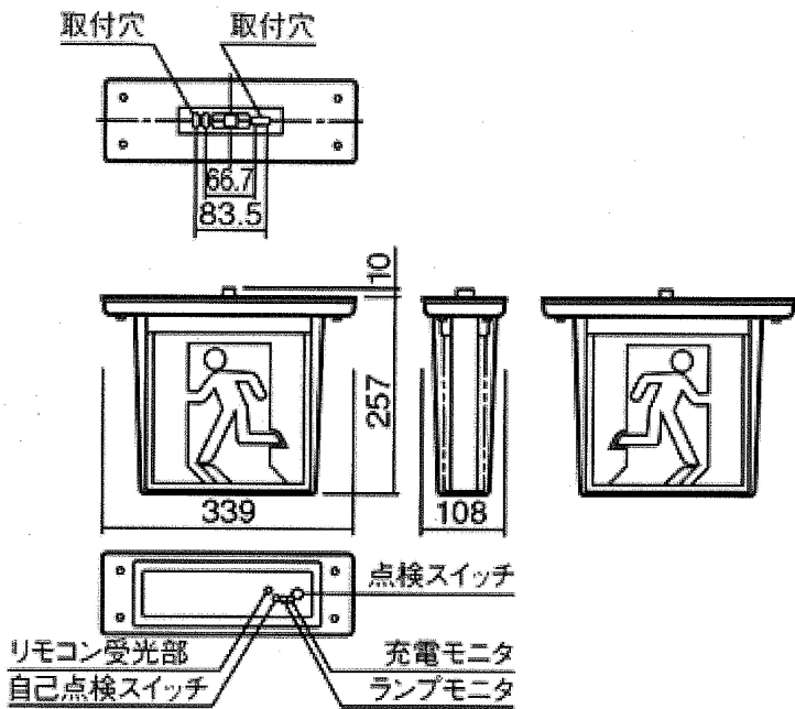
誘導灯B級B.L形両面（天井吊下げ型）参考図
