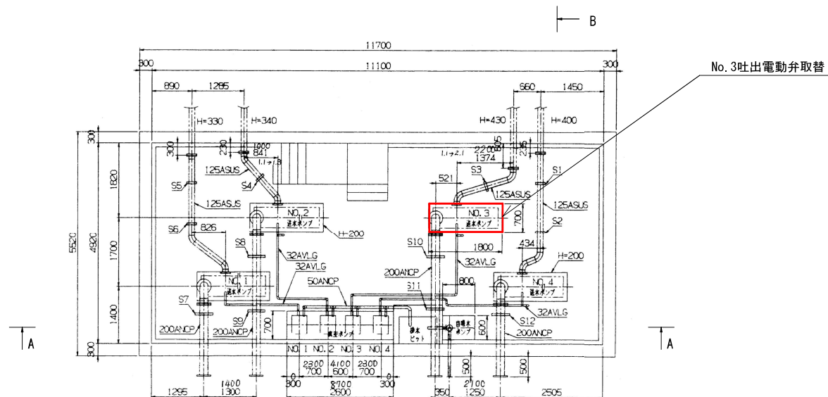
地下1階ポンプ室平面図 S=Free
