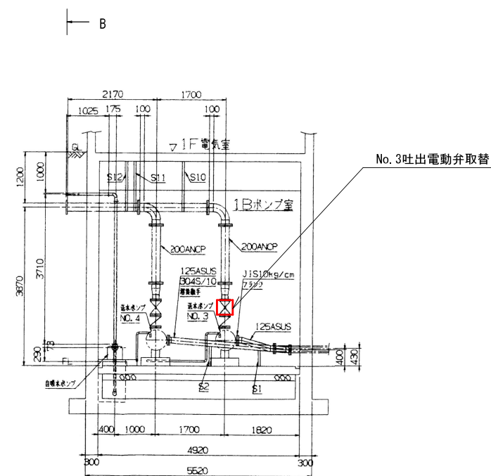
B-B断面図 S=Free
