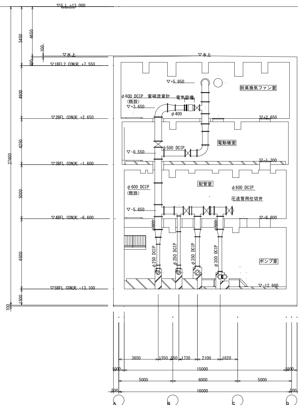
B-B断面图
