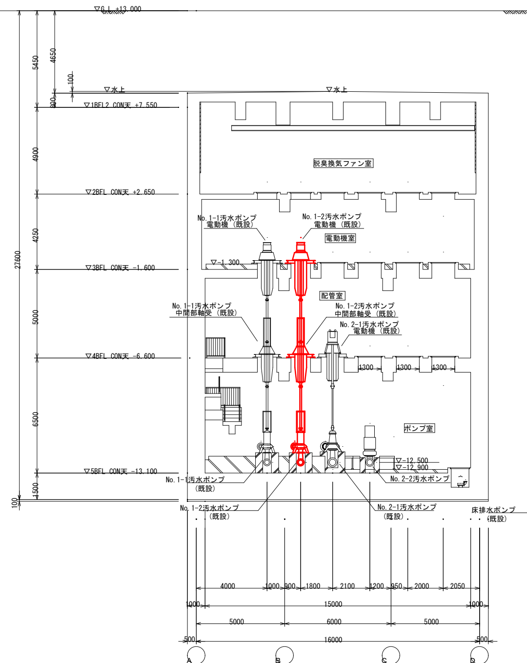
C—C断面図
