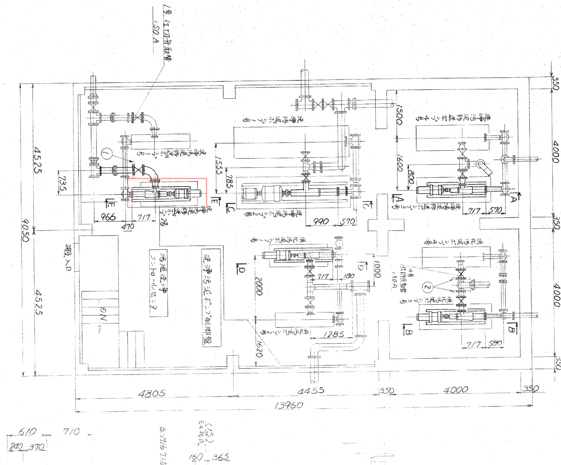
洗浄汚泥移送ポンプ配置平面図
