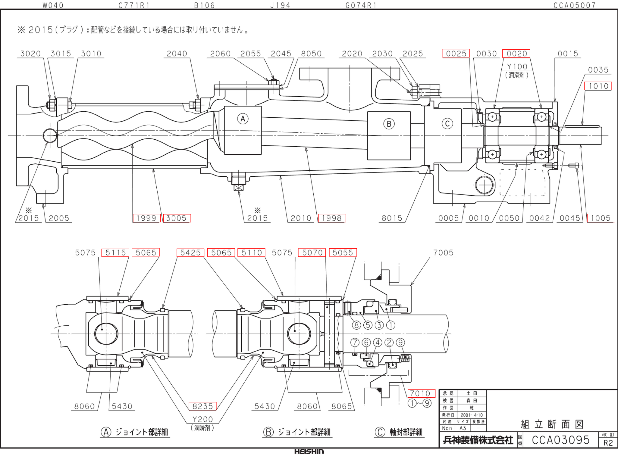
洗浄汚泥移送ポンプ組立断面図
