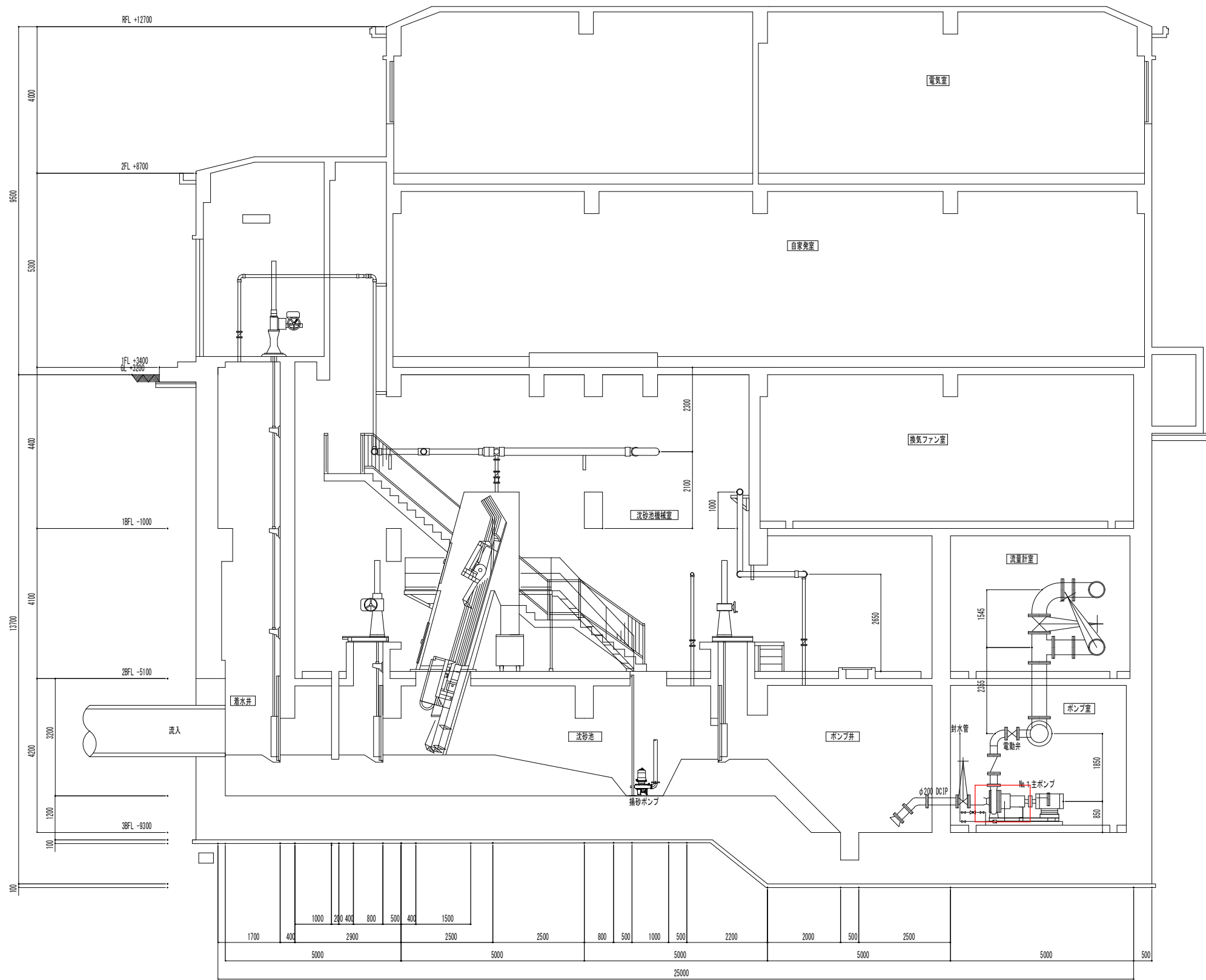
武久中継ポンプ場断面図
