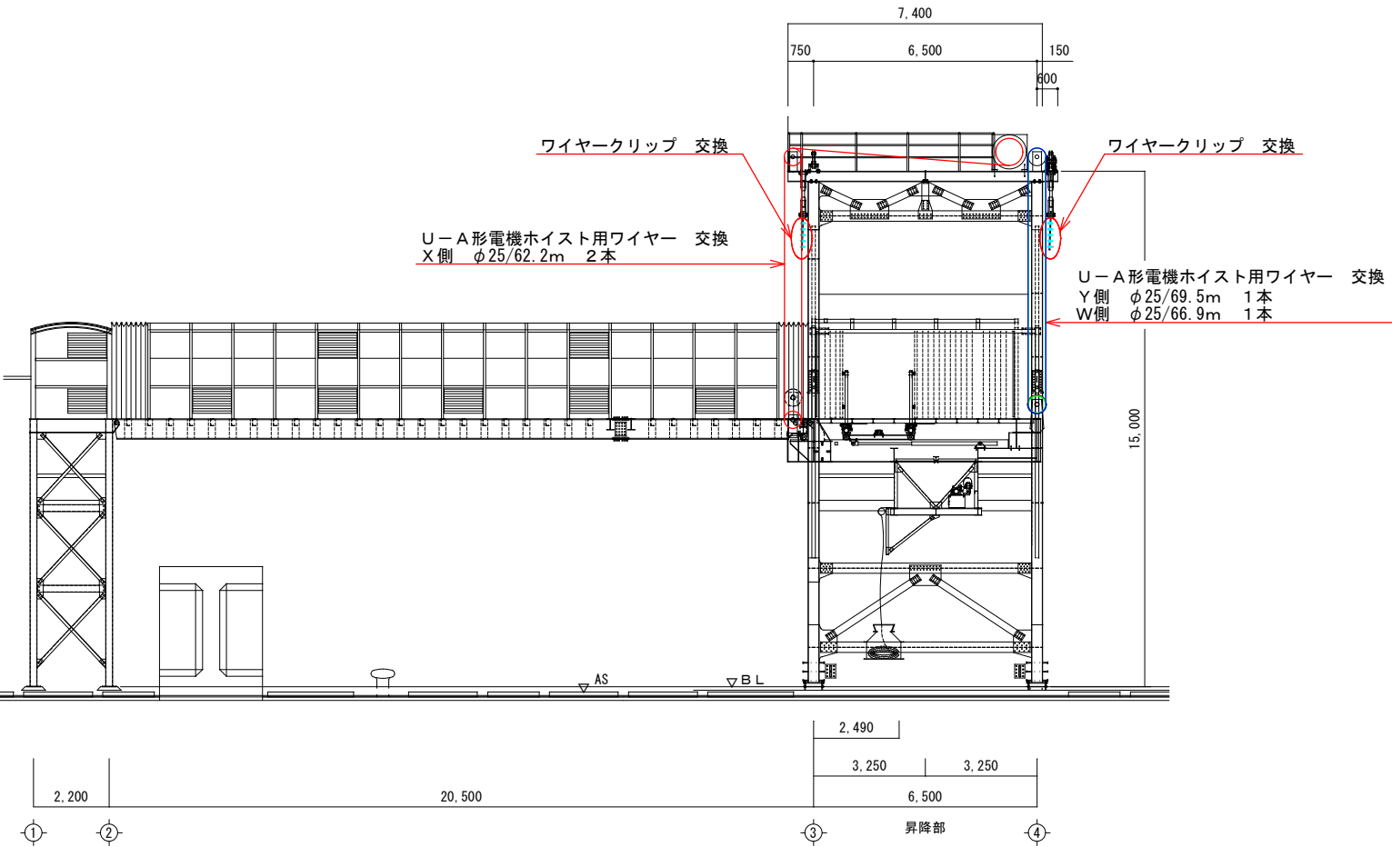
断面図 S=1:FREE
