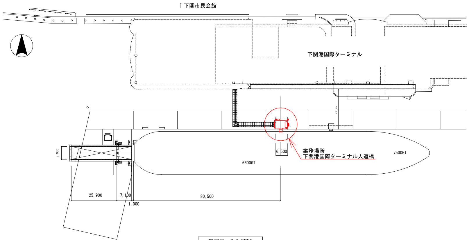
配置図 S=1:FREE
