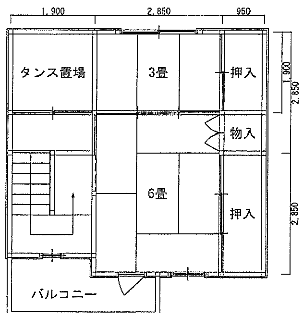
2階平面図
