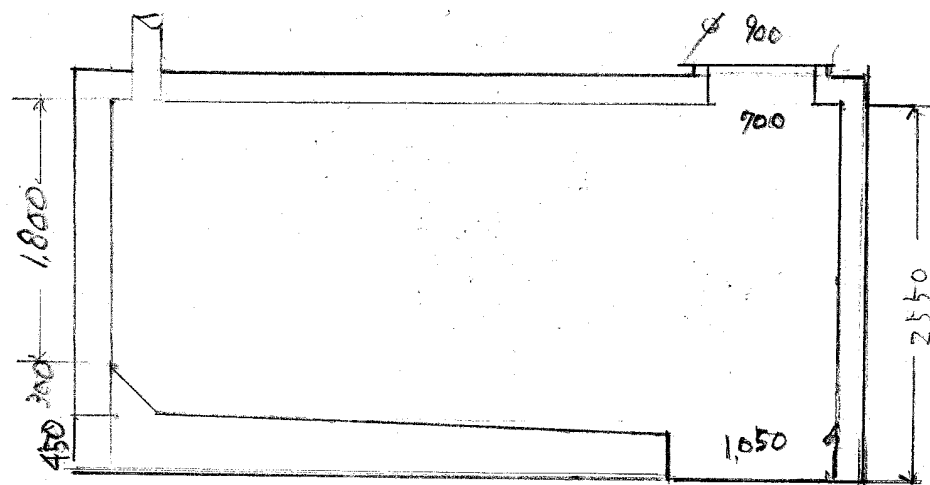
立面図
