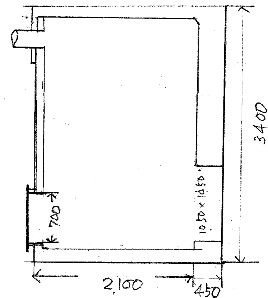
断面図
