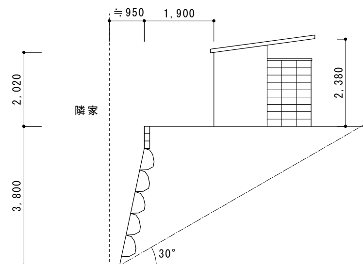
敷地断面図 S=1:100
