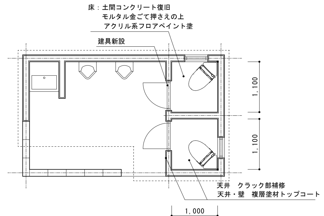
改修後平面図 S=1:50
