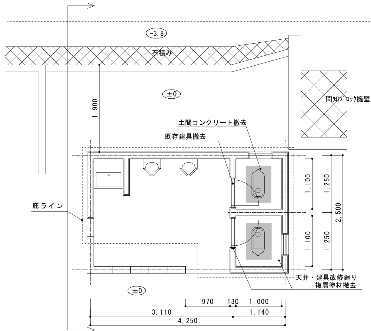
既存平面図 S=1:50
