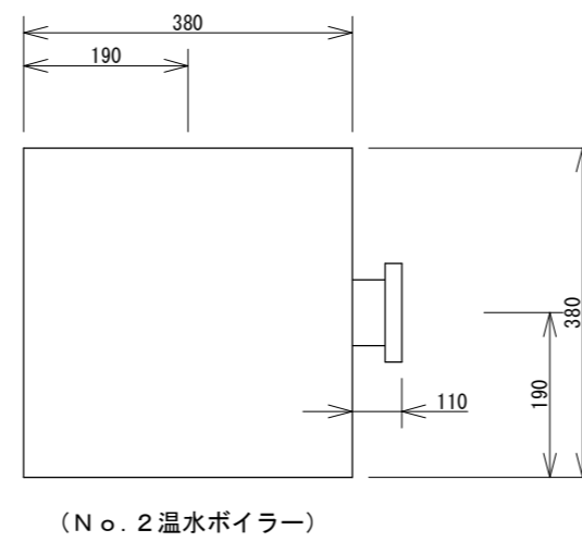
測定位置断面図 S: Free
