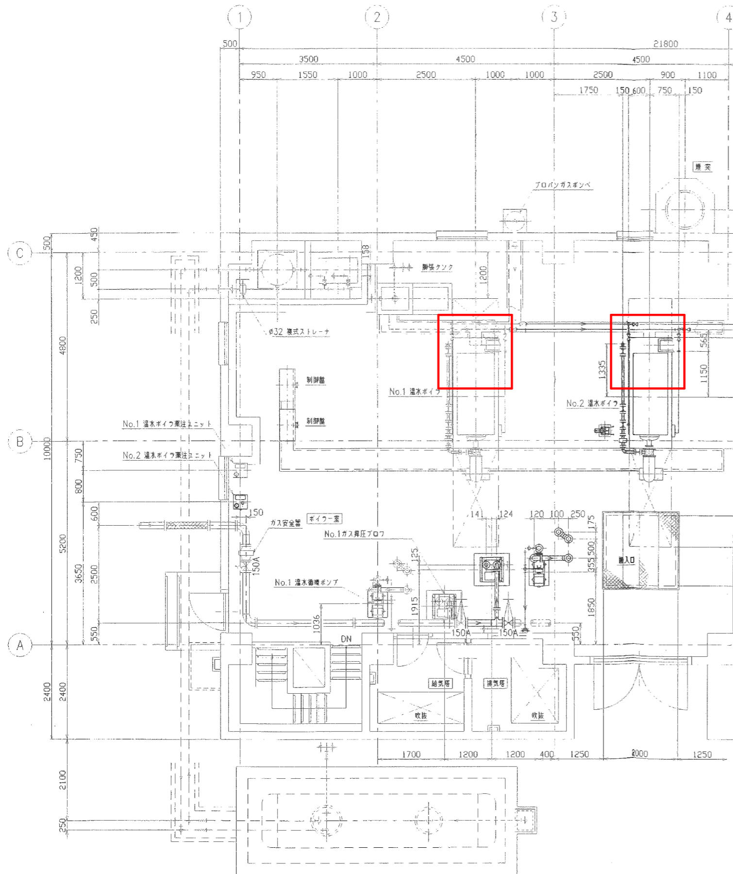
ボイラー室平面図 S: Free
