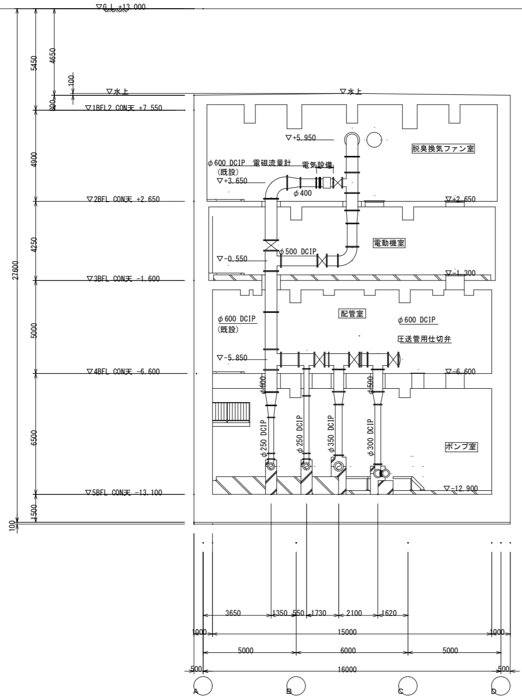
B-B断面図
