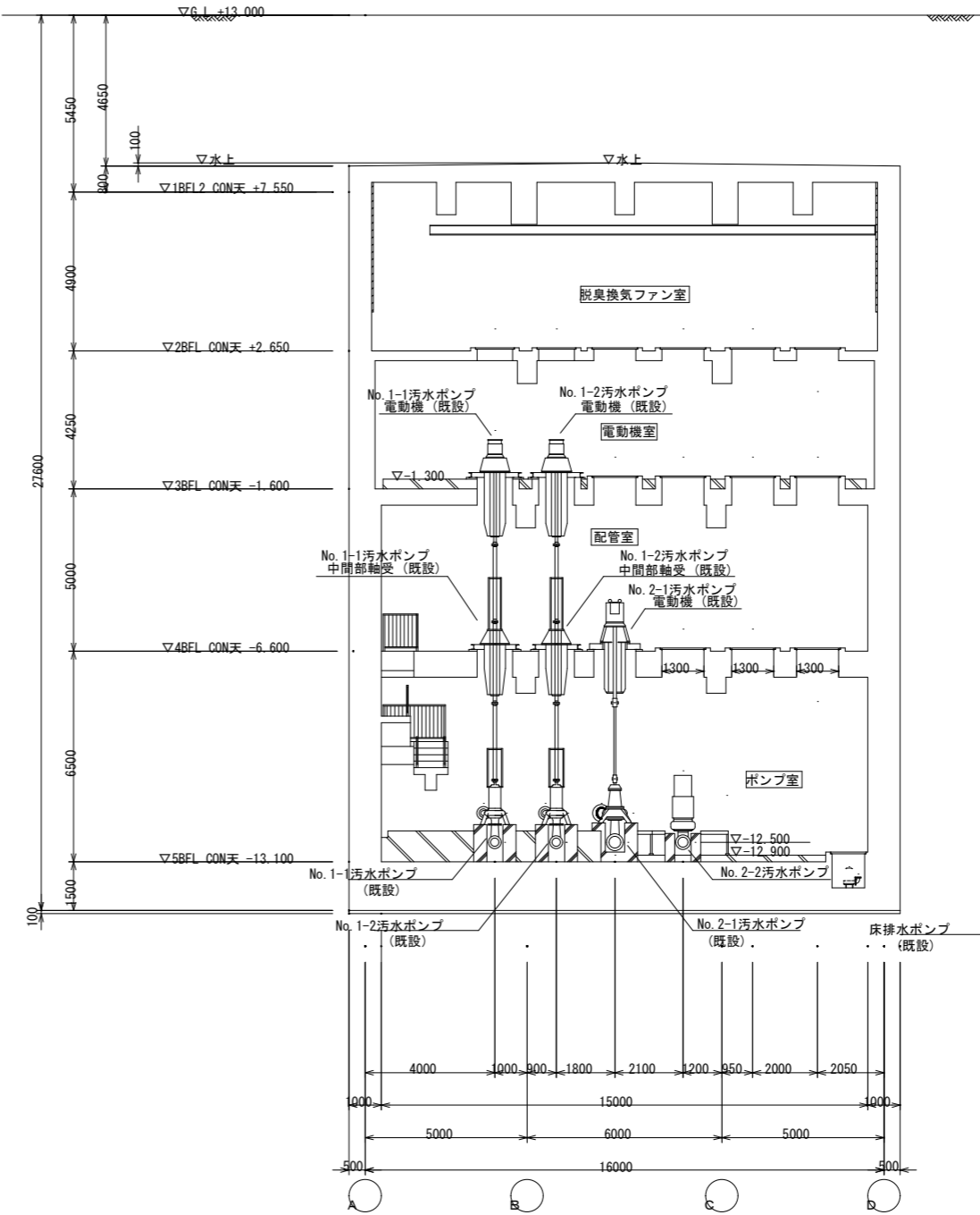
C-C断面図
