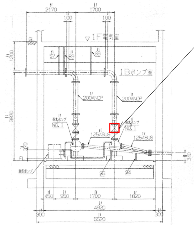
B-B断面図 S=Free
