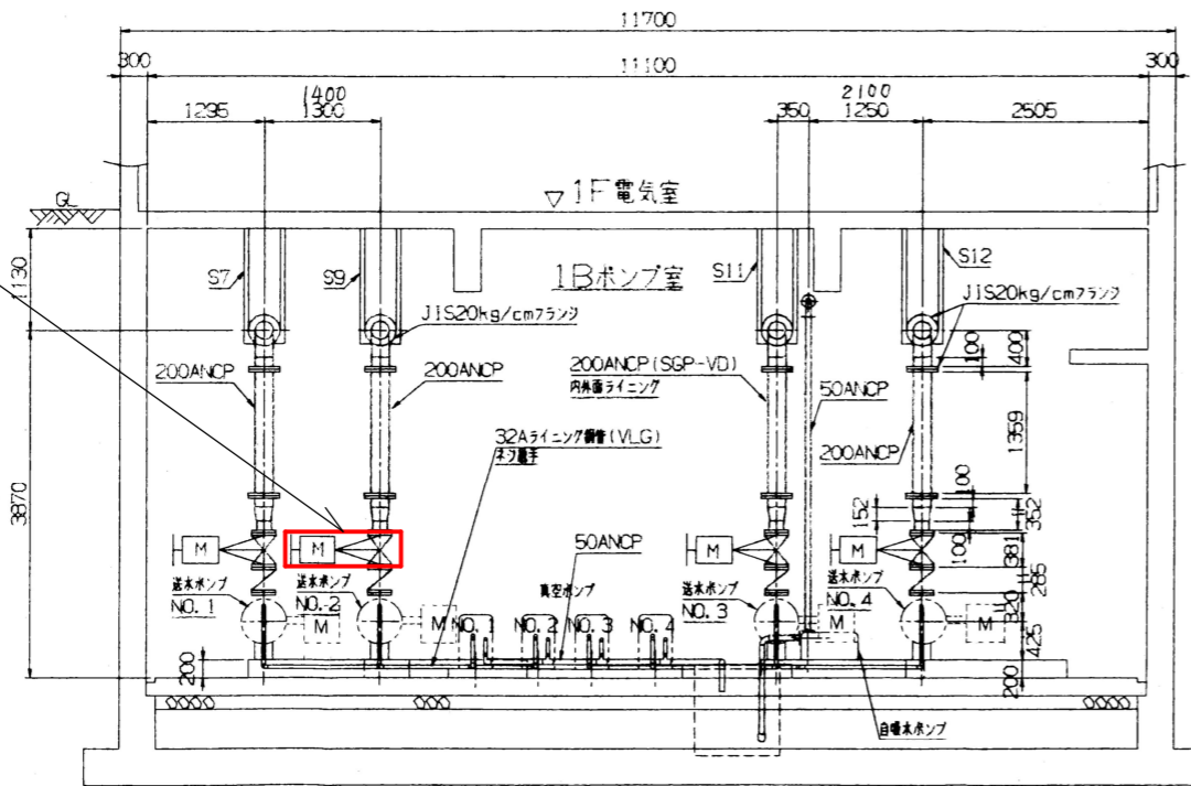
A-A断面図 S=Free
