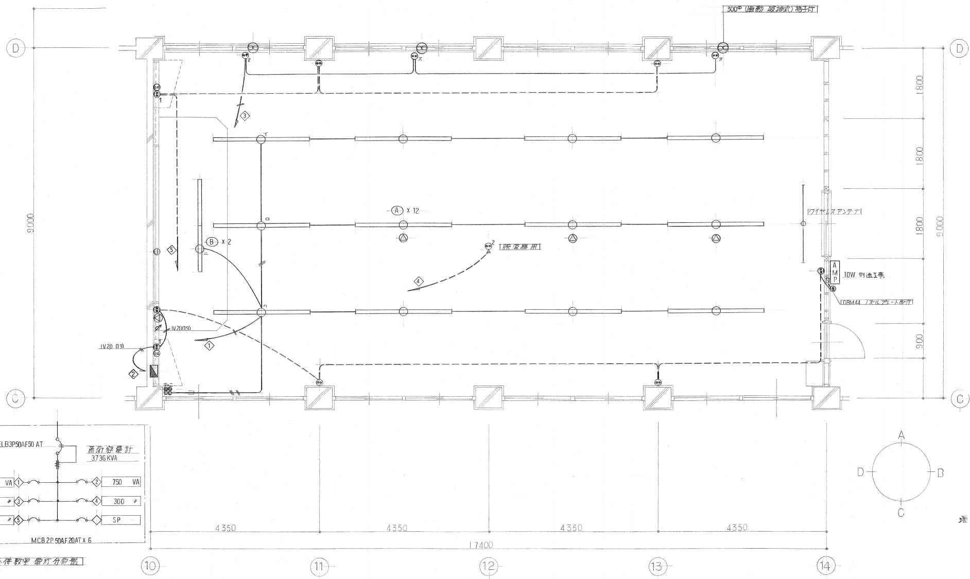
2F 合併教室 平面 図 S=1:50
