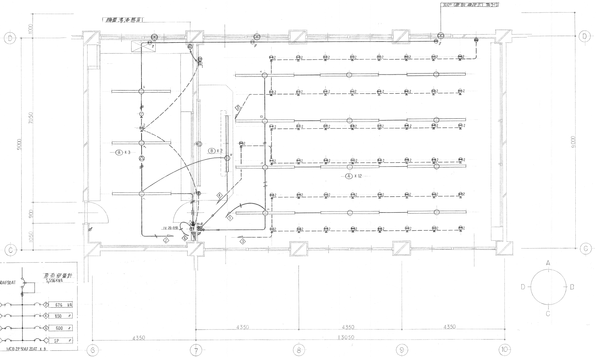
3F英文タイト電平面図 S=1:50
