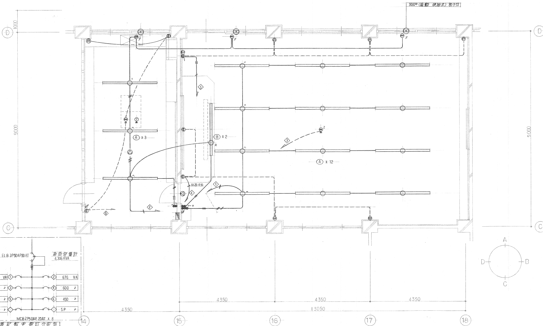
3F 海記教室 平面 圖 S=1:50
