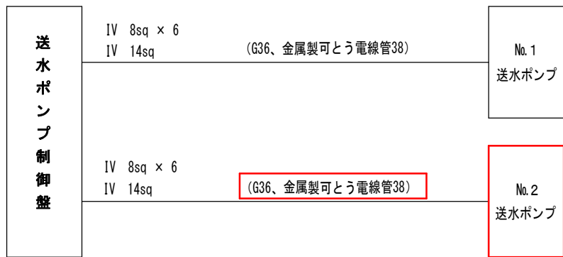
配線系統図
