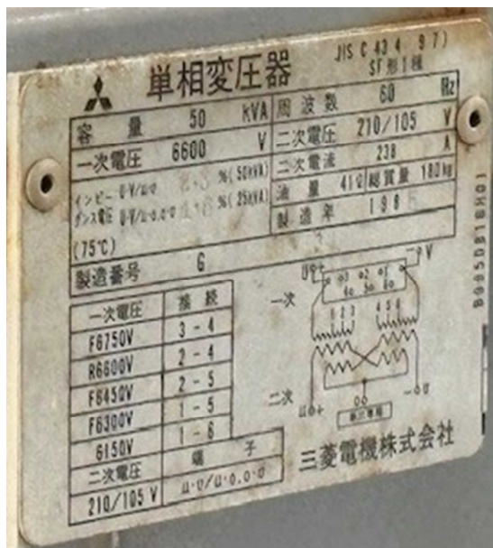
受電設備
