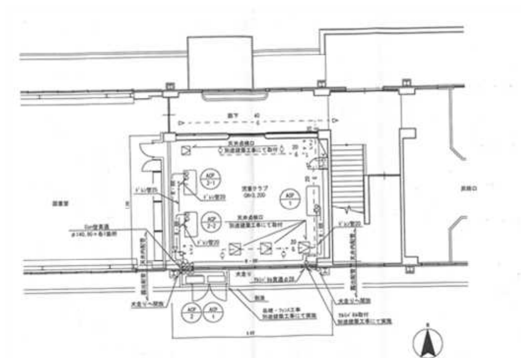
平面図②（既設空調機設置時） （川中③児童クラブ）
